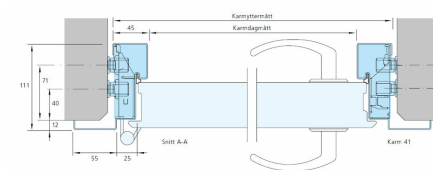
Skiss enkeldörr, snitt A-A.
